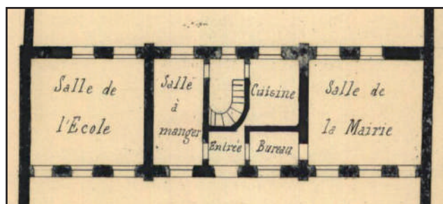
Plan du rez-de-chaussée, 1899 ©AD78 1T mono 1/10
